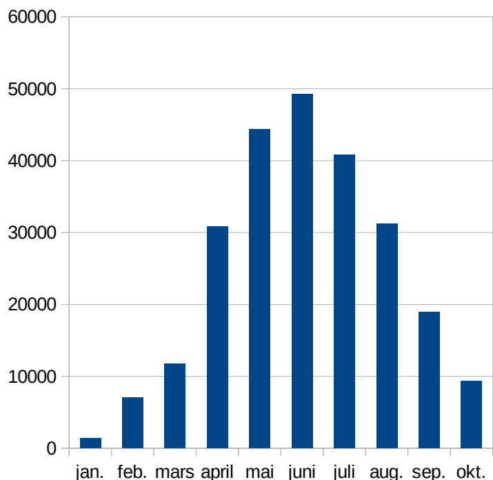
Solcelleproduksjon i år: 245 000 kWh
